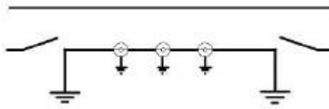
Slika 13. Rad na jednom stupu (srednjem) dvosustavnog voda
